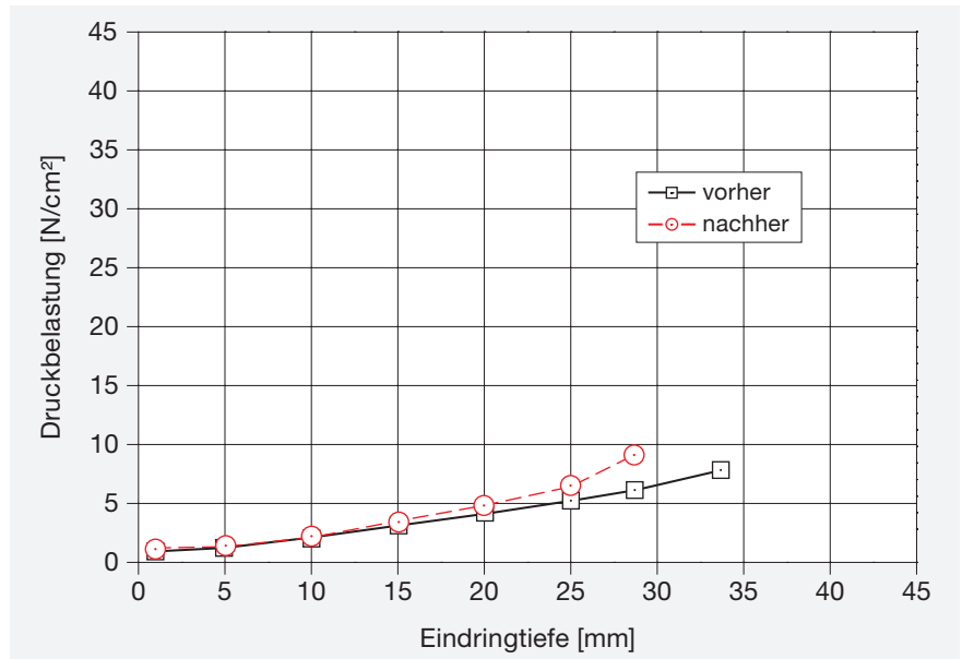
Bild 4: Verformbarkeit in Abhängigkeit vom Auflagedruck vor und nach der Dauertrittbelastung
